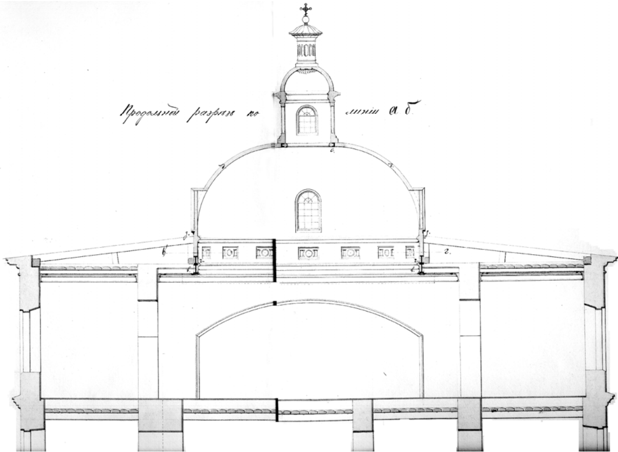
Проект на постройку купола церкви. ГАПО. Ф. 198. Оп. 1. Д. 372. Л. 322.
